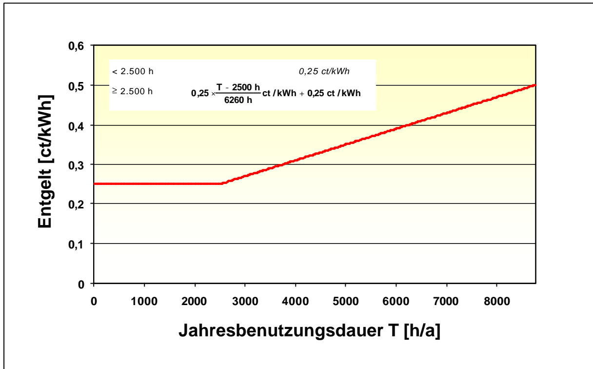
Bild 1: Vermiedene Netznutzungsentgelte bei dezentraler Einspeisung in Niederspannung ohne registrierende Leistungsmessung (Beispiel)
